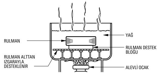
Şekil 10. Isıyla genişletirme yöntemi.
